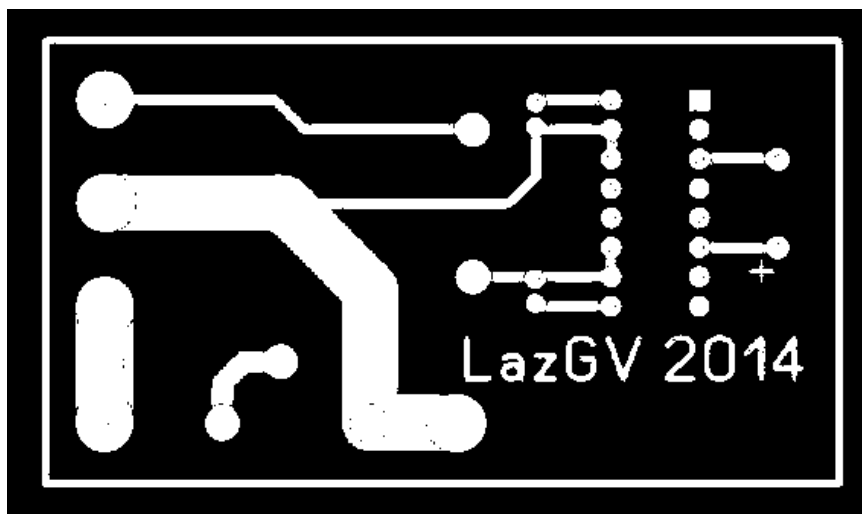
Рис. 3. Печатная плата регулятора мощности
