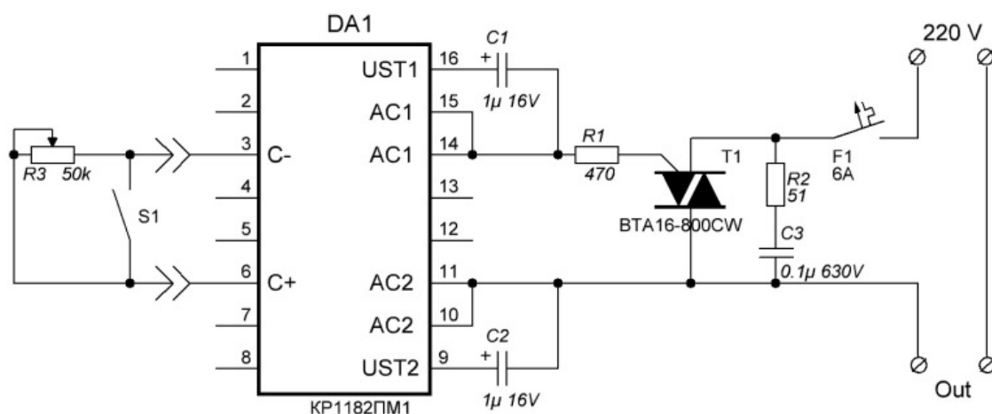
Рис. 2. Схема регулятора мощности
