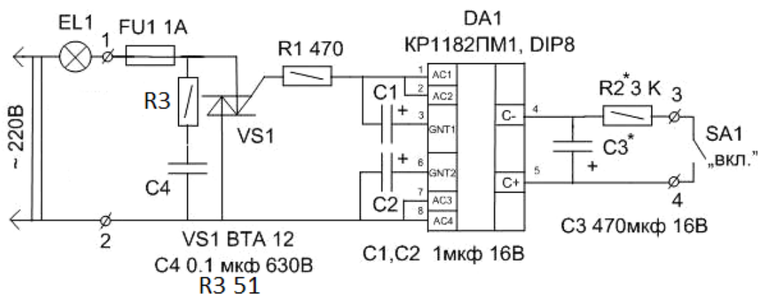
Рис. 1. Схема устройства плавного включения ламп накаливания
